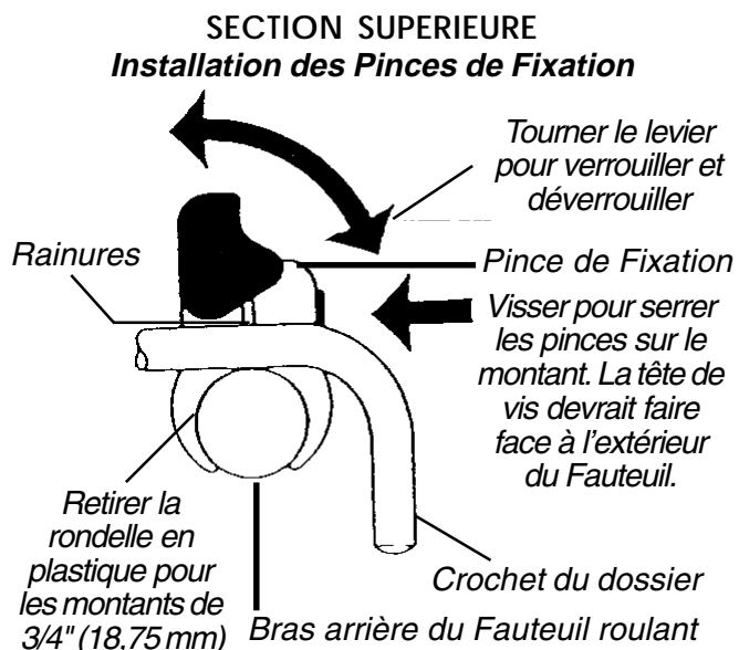
Vue du haut - montant droit du fauteuil roulant SCHEMA 1 - INSTALLATION DE ULTI-MATE AIR BACK SUR LES MONTANTS DE DOSSIER
